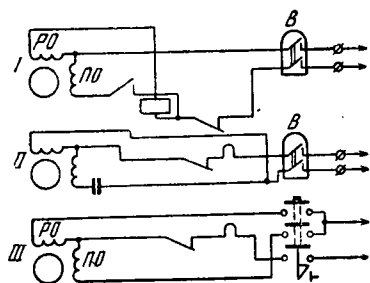
Рис. 1. Электрические схемы стиральных машин типа СМР-1,5 (наиболее типичные):
