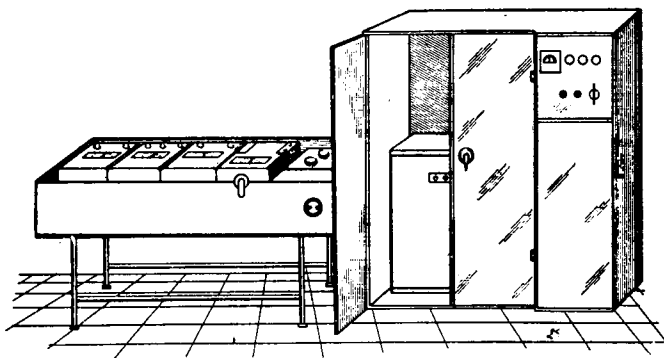
Рис. 28. Рабочее место для испытания стиральных машин после ремонта
