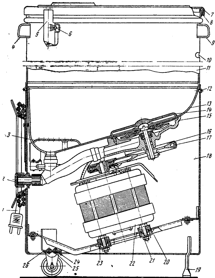
Рис. 3. Стиральная машина «Рига-8»:
