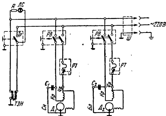
Рис. 18. Электрическая схема стиральной машины «Аурика-71п»:
