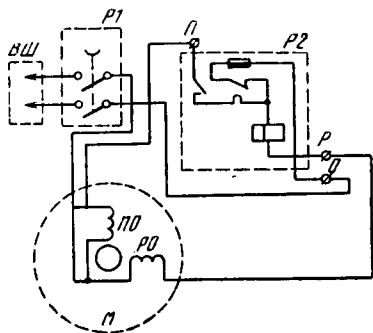
Рис. 6. Электрическая схема стиральной машины «Волга-8 м»:
