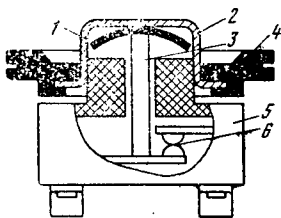
Рис. 17. Датчик температуры:
