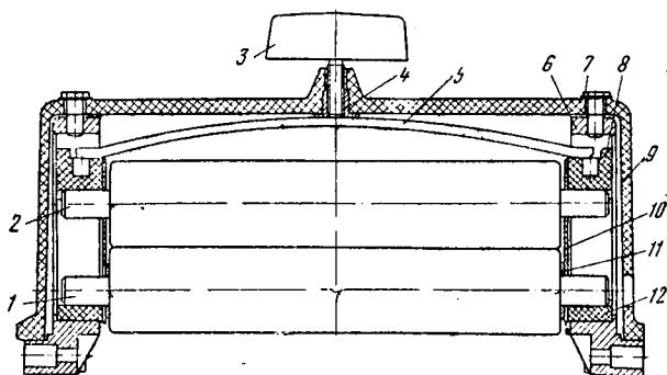
Рис. 7. Отжимное устройство стиральной машины СМР:
