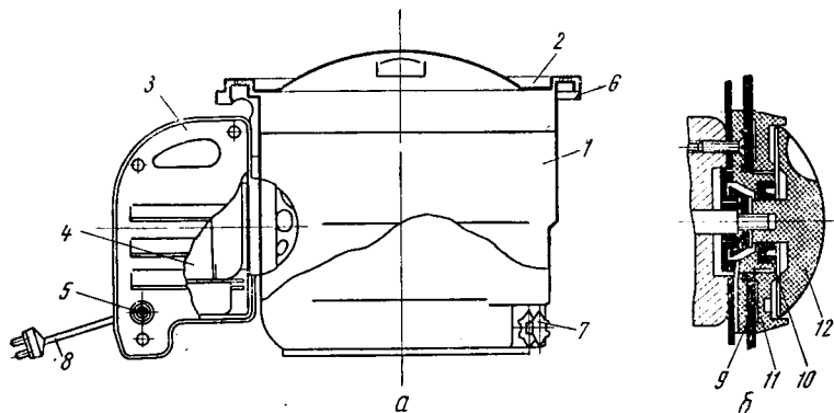
Рис. 2. Стиральная машина «Малютка-2»:
