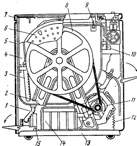
Рис. 19. Стиральная машина «Снежинка»:
