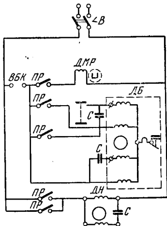
Рис. 20. Электрическая схема стиральной машины «Снежинка»:
