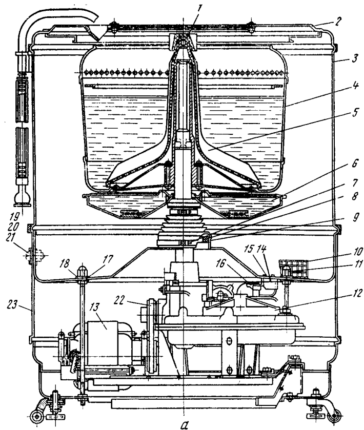
Рис. 21. Стиральная машина
