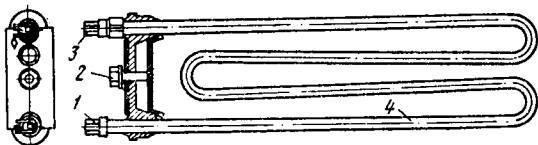
Рис. 16. Электронагреватель стиральной машины «Аурика-71п»:
