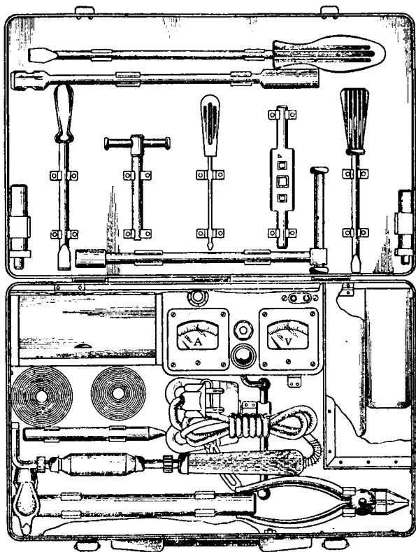
Рис. 29. Переносный комплект инструмента для ремонта стиральных машин
