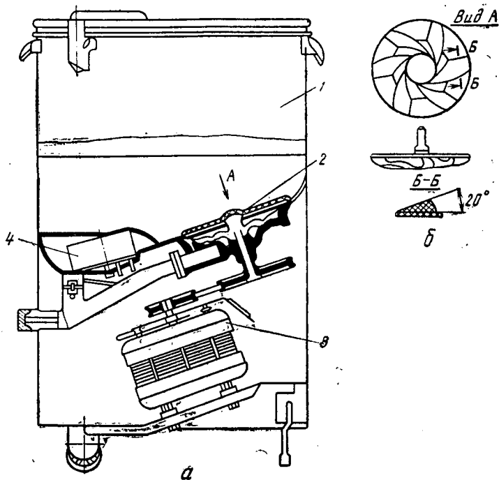
Рис. 4. Стиральная машина «Рига-12»:
