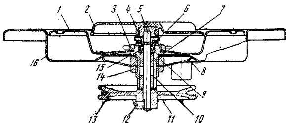
Рис. 12. Узел активатора:
