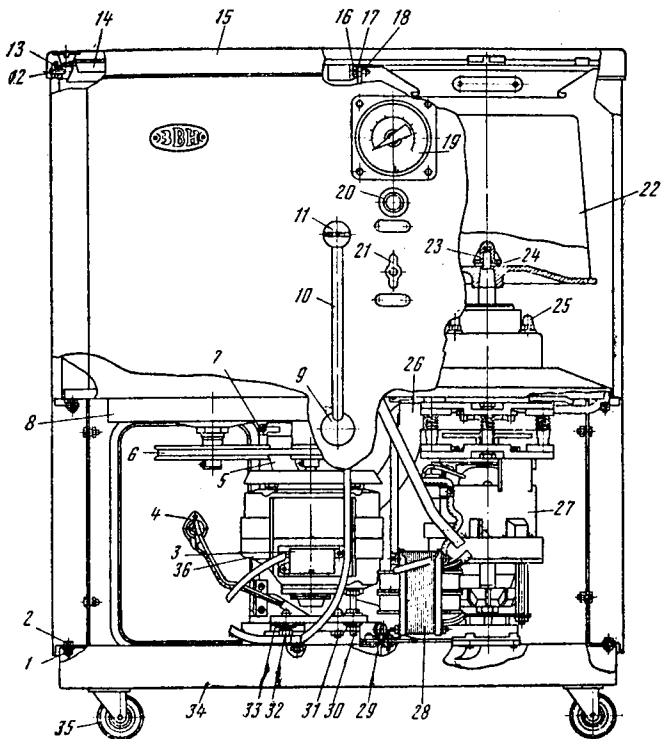
Рис. 11. Стиральная машина ЗВИ:
