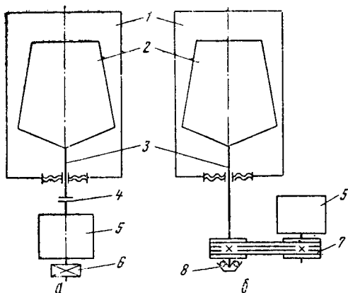
Рис. 9. Принципиальные схемы конструкции узла centrifуги полуавтоматических стиральных машин:
