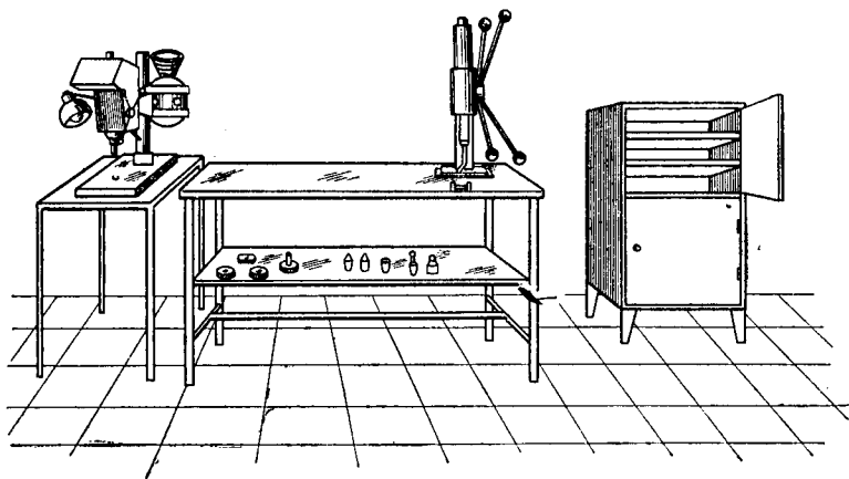
Рис. 27. Рабочее место для ремонта узлов стиральных машин
