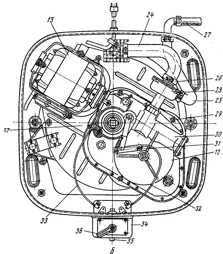
УСМ-1 «Харьков»:
