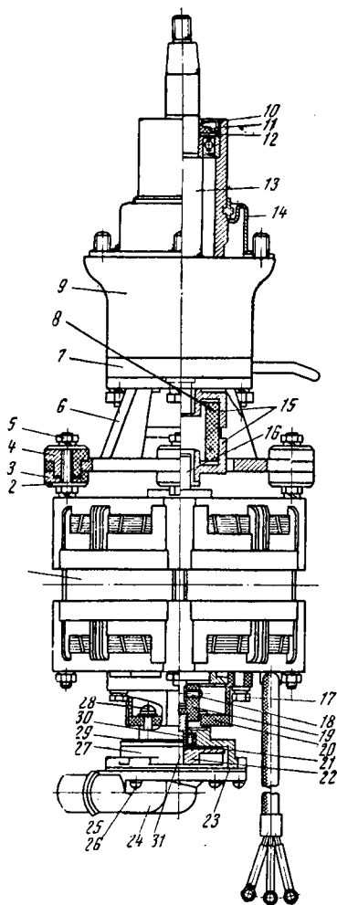
Рис. 14. Узел центрифуги с электродвигателем типа ДАО-ц:
